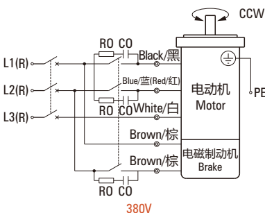
380V
