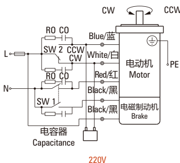
220V
