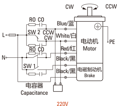
220V
