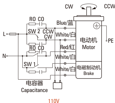
110V
