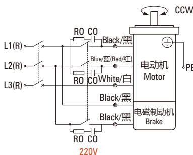
220V
